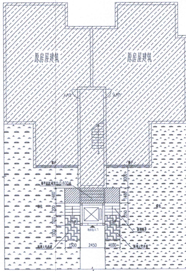
增设电梯一层示意图 1:100
