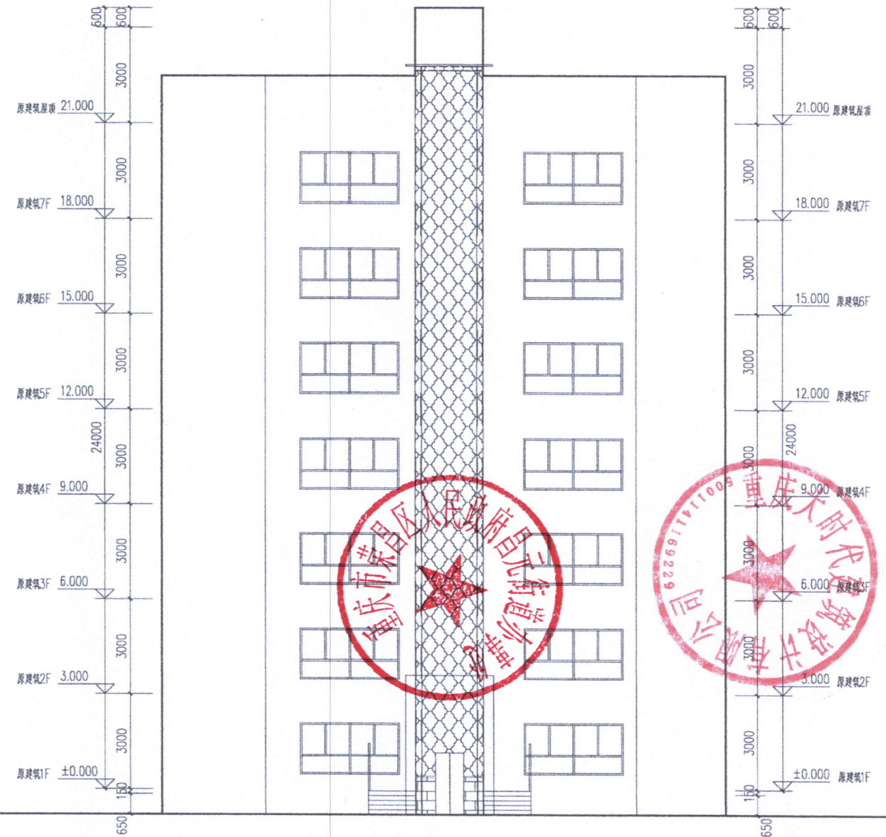
增设电梯立面示意图 1:100
