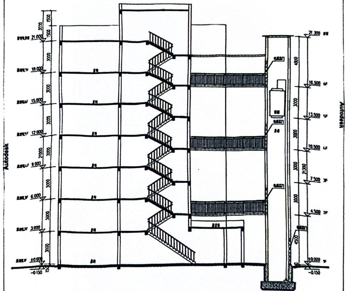
增设电梯剖面示意图 1:100
