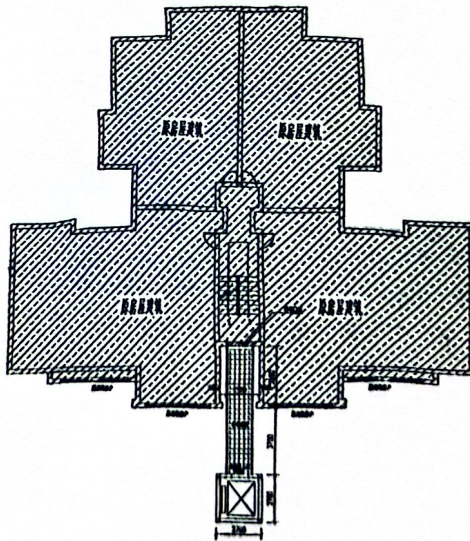
增设电梯一层示意图 1:100
