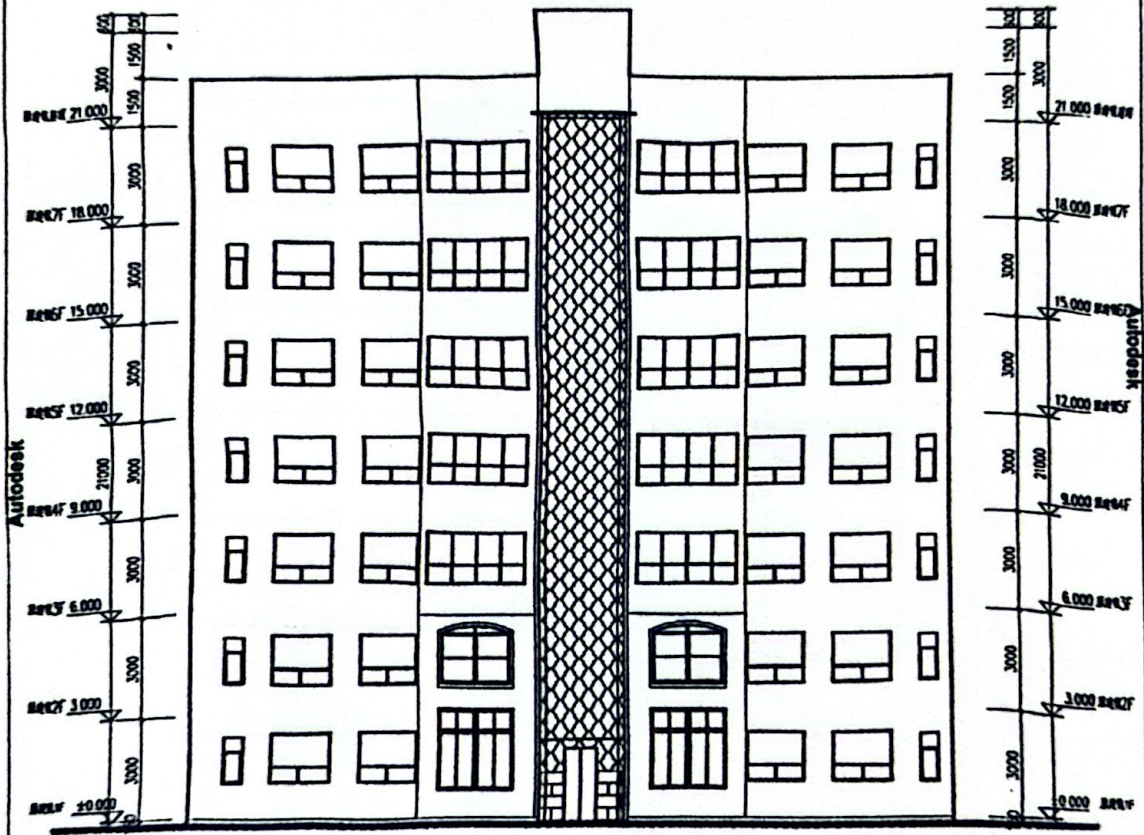
增设电梯立面示意图 1:100
