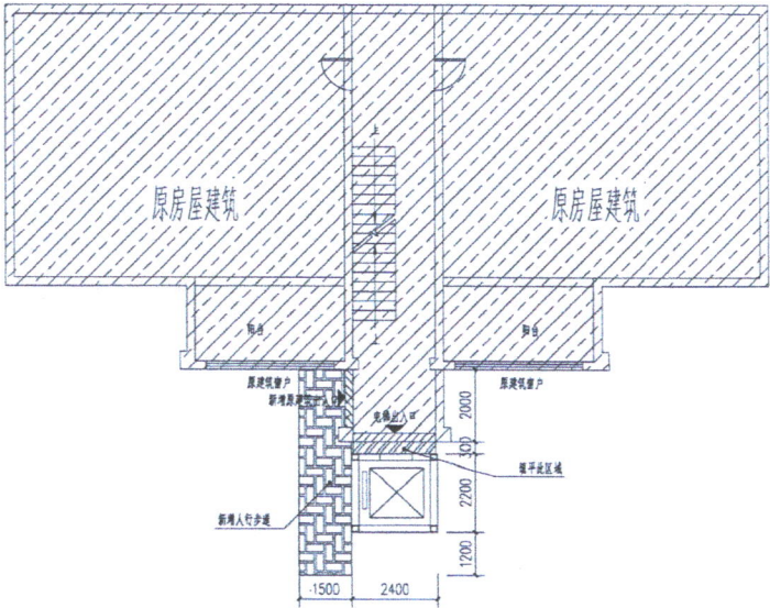
增设电梯一层示意图 1:100
