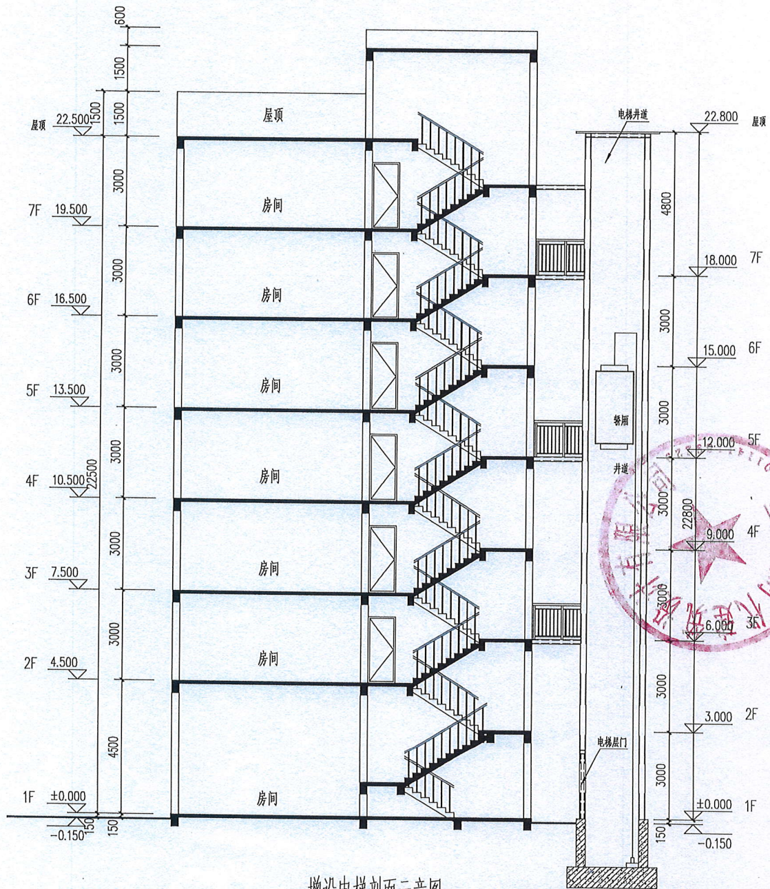
增设电梯剖面示意图 1:100
