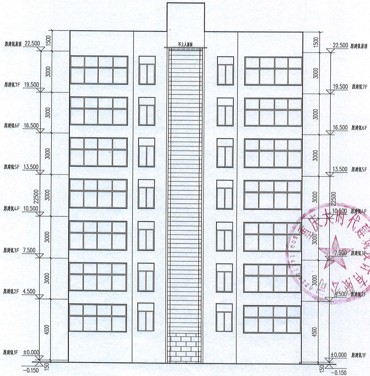
增设电梯立面示意图 1:100
