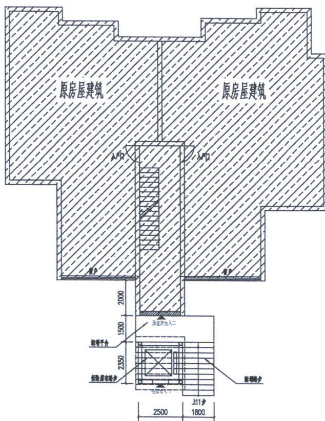
增设电梯一层示意图 1:100
