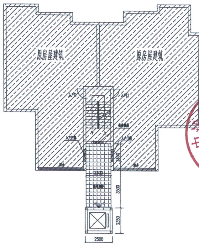
增设电梯标准层示意图 1:100
