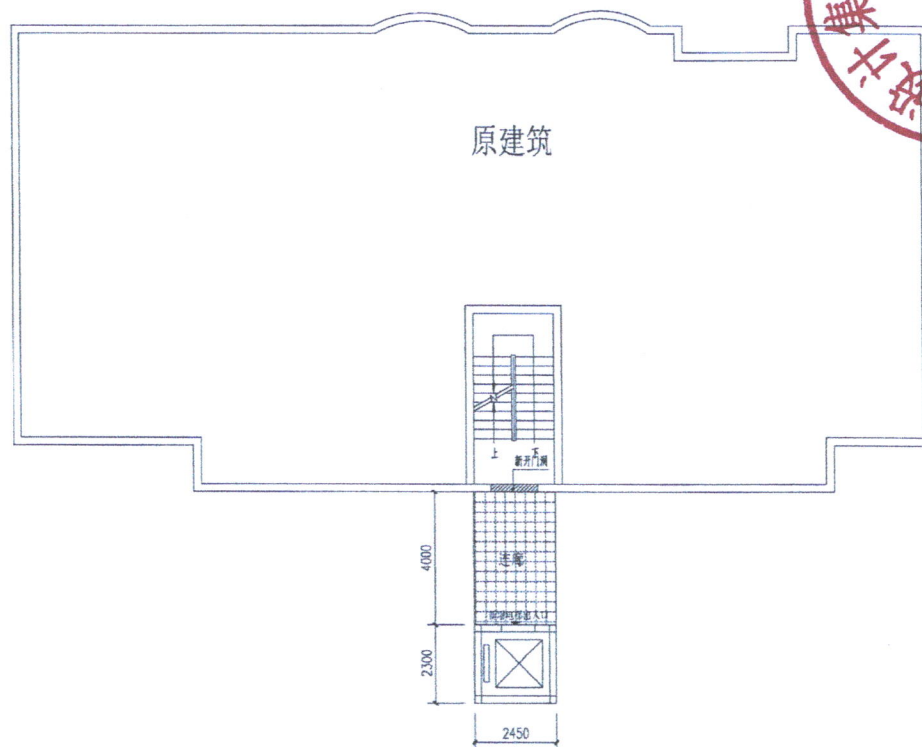
标准层平面示意图 1:100
