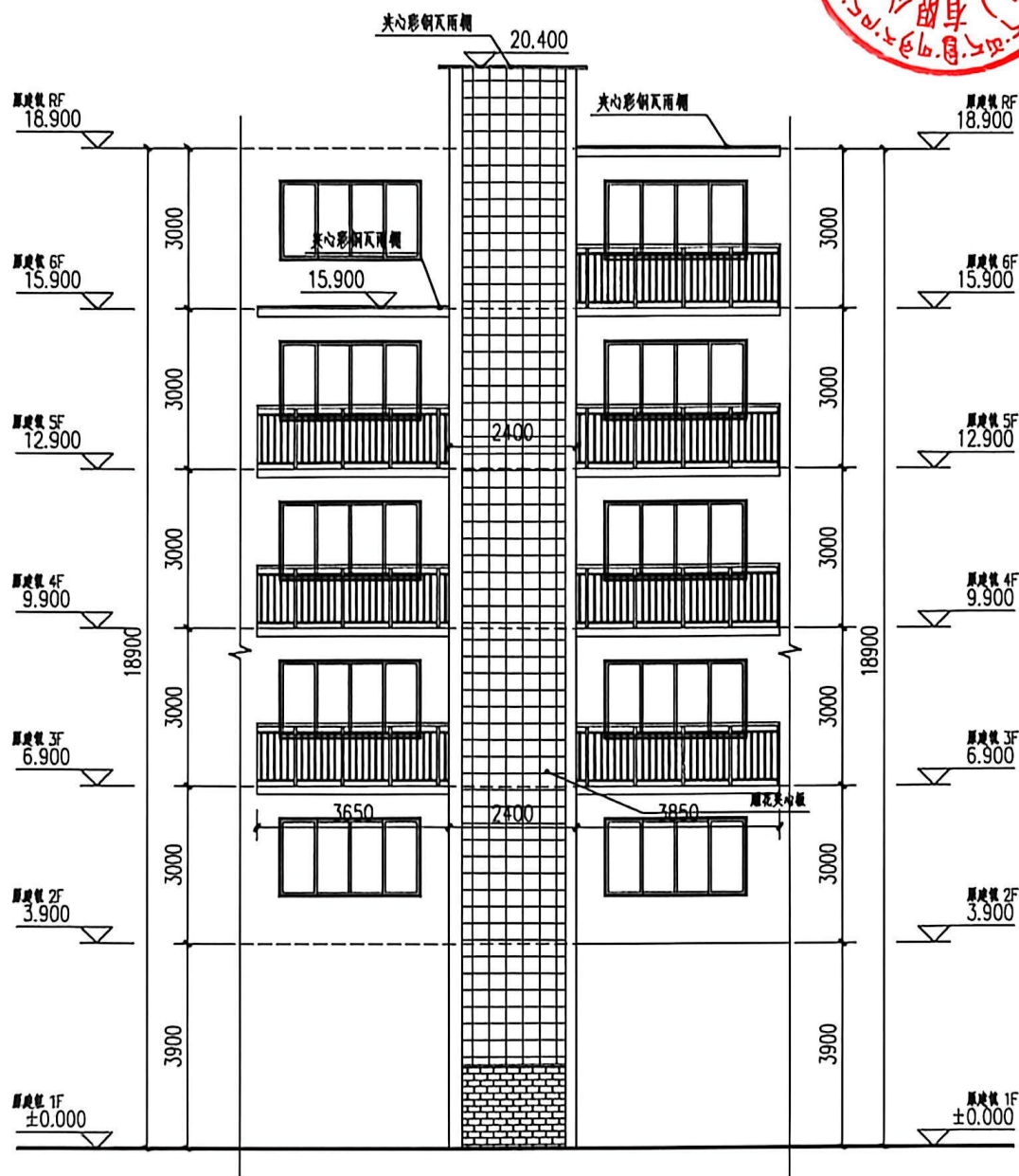
增设电梯立面示意图
