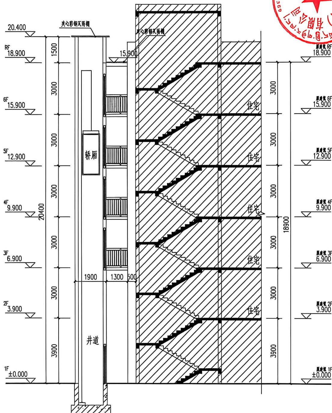
增设电梯剖面示意图
