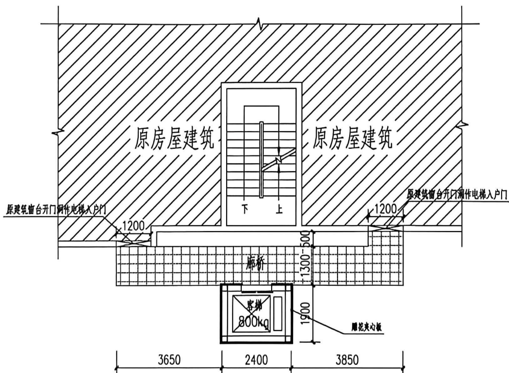
增设电梯一层平面示意图
