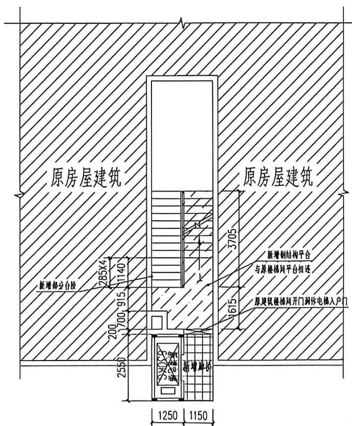
增设电梯标准层平面示意图
