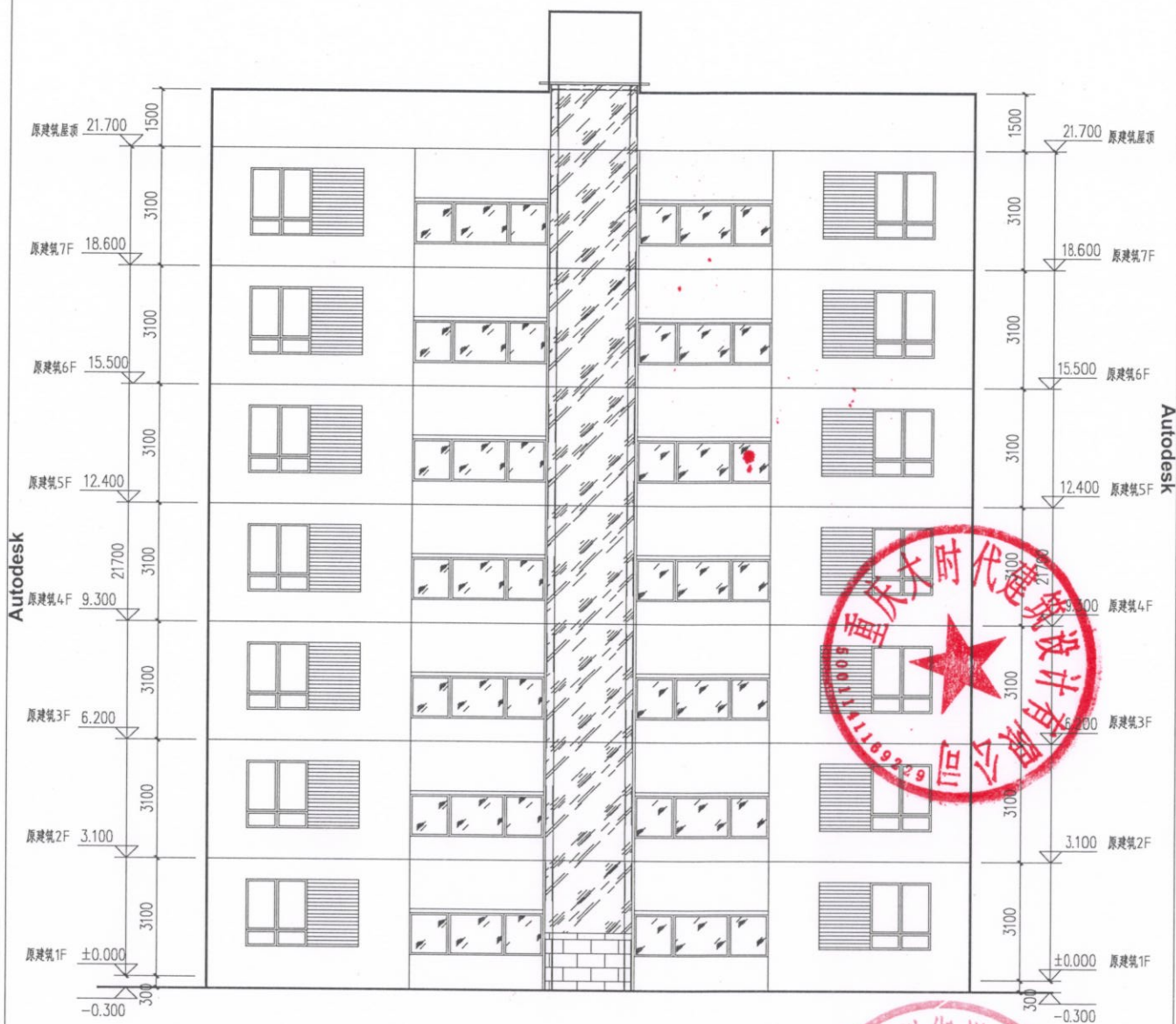
增设电梯立面示意图 1:100
