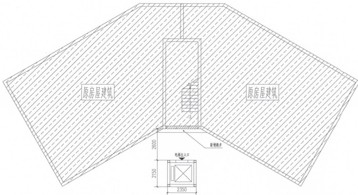
增设电梯一层示意图 1:100
