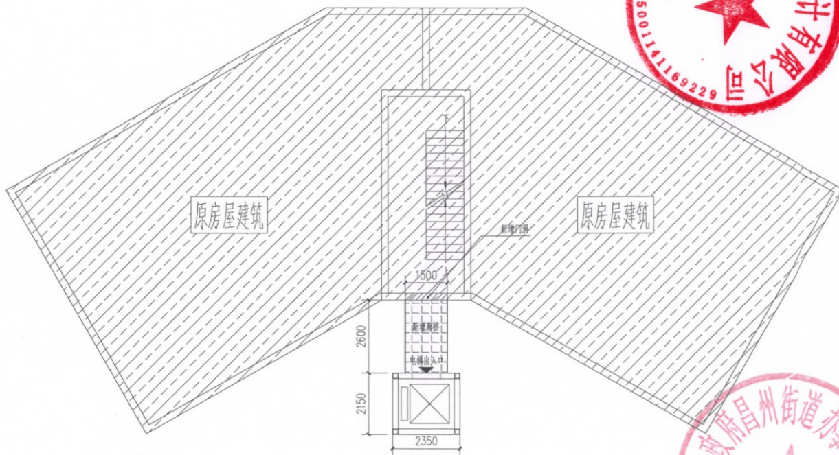
增设电梯标准层示意图 1:100
