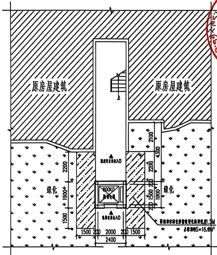
增设电梯首层平面示意图
