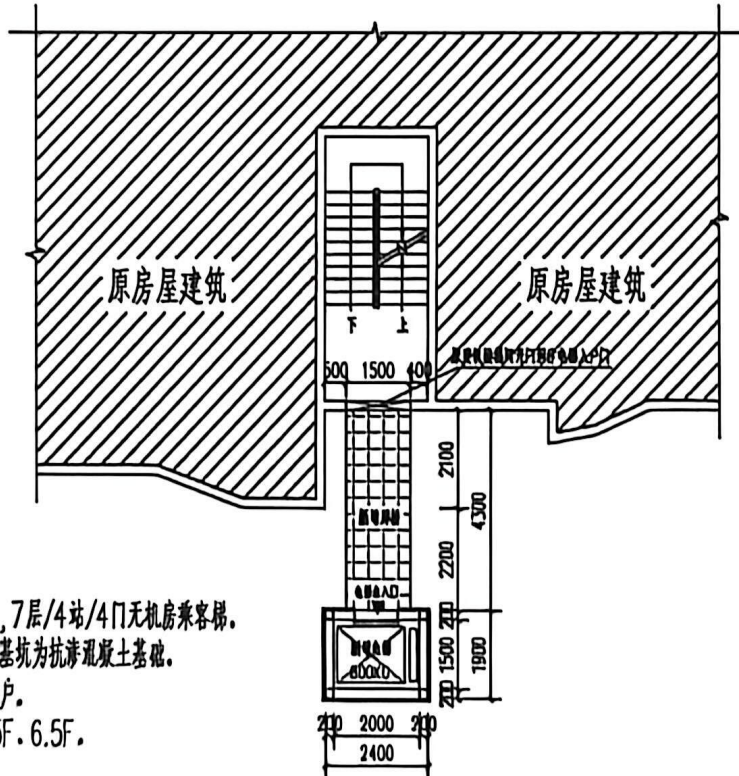
增设电梯标准层平面示意图
